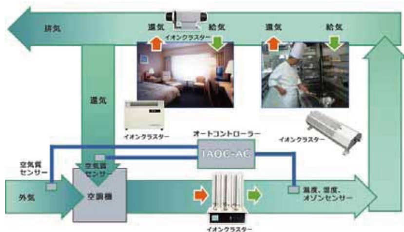
IAQC-DUCT (建物空調用清浄システム)ビル内設置イメージ
